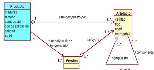
Figura 2. Diagrama de la subontología de los productos
